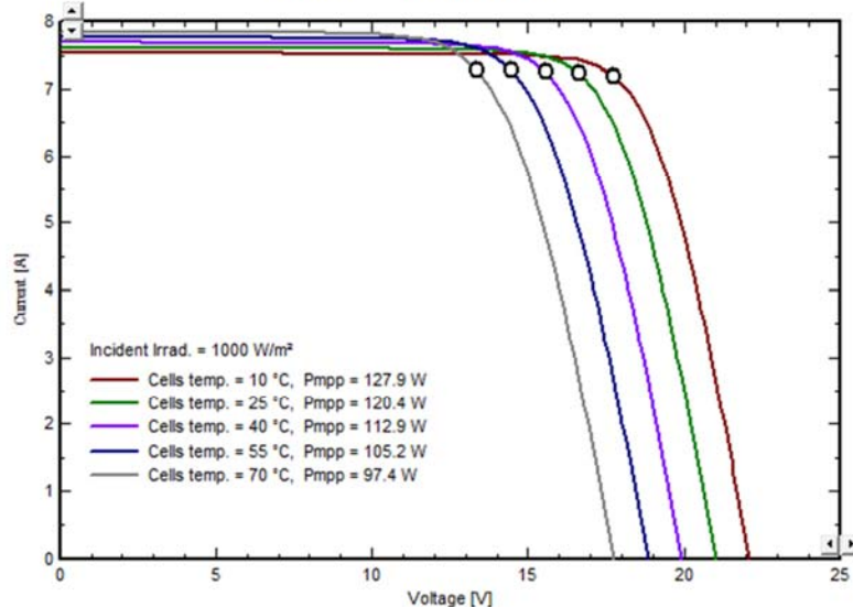
PV module: Waaree, WS-120
