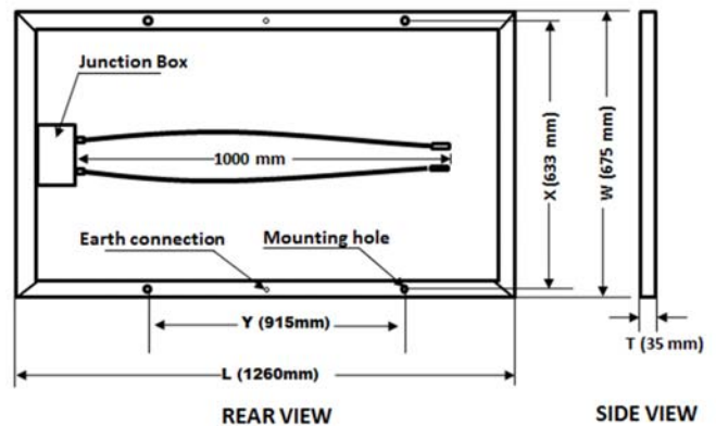
PV module: Waaree, WS-120
