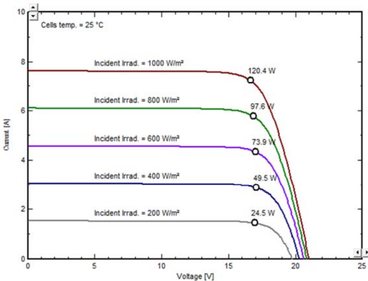
PV module: WAAREE, WS-120
